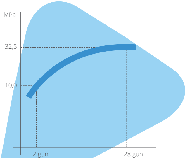
Basıncı Dayanımı Gelişim Eğrisi · Minimum Değerler
